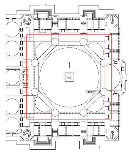
Edirne, a Szelim-mecset. Szinán 1568 és 1575 között építette. A kupola átmérője 31,3 m, magassága 71 m.
